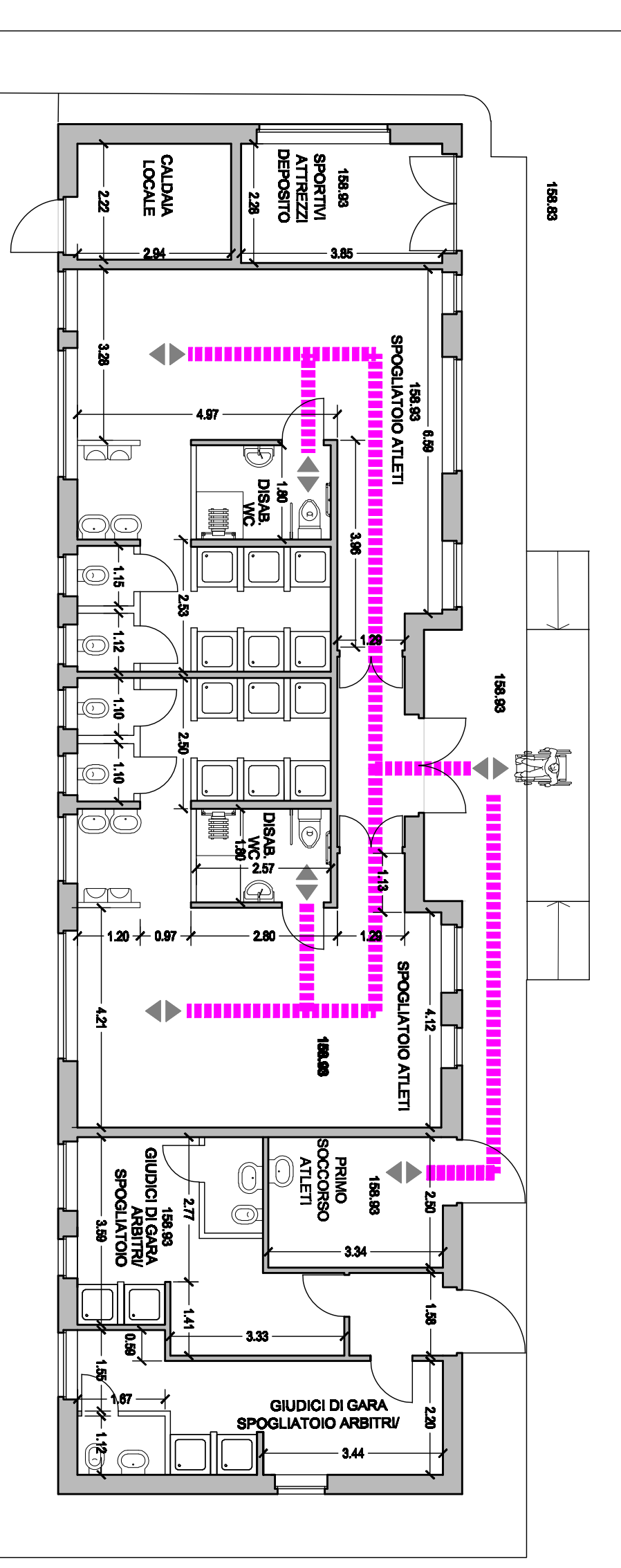
PIANTA BLOCCO SPOGLIATOI ATLETTI/ADDETTI scala 1:100
