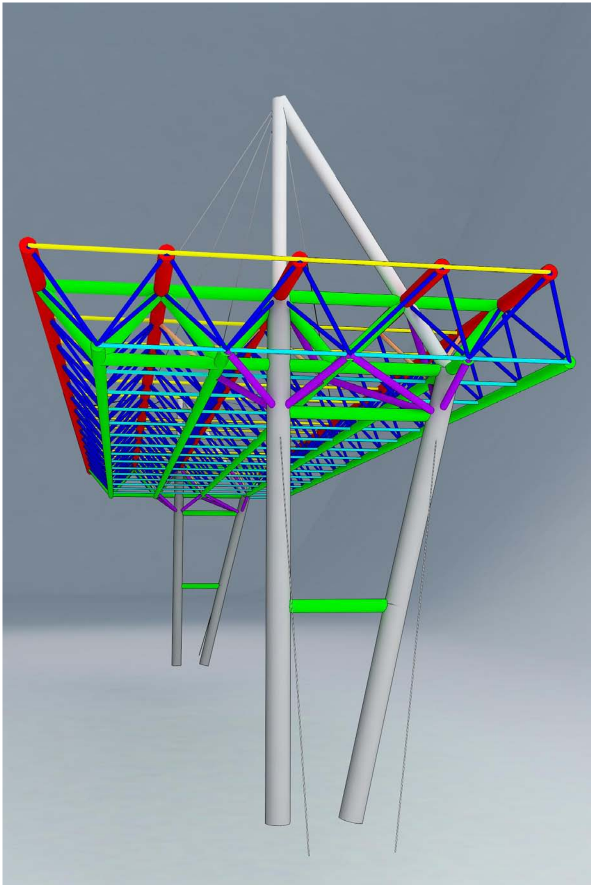
DETTAGLIO STRUTTURALE COPERTURA TRIBUNA
